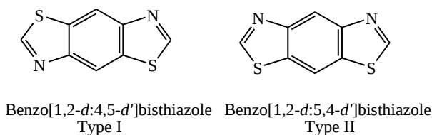
Fig. 1. Linear Benzobisthiazoles
