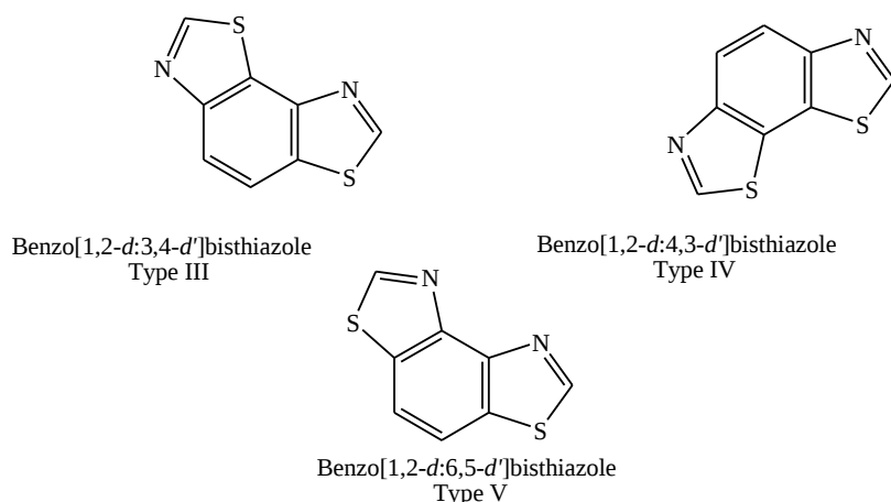
Fig. 2. Angular Benzobisthiazoles
