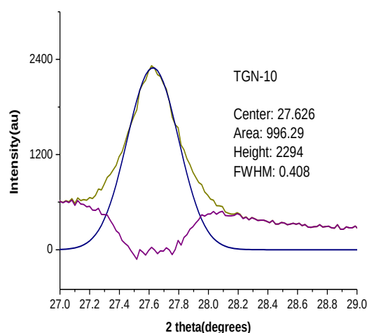
Figure (5): Fityk analysis for TGN-10
